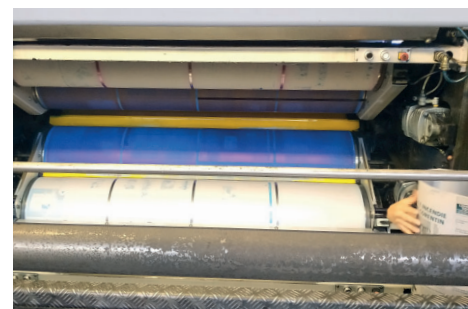
Ici le rouleau avec les plaques en aluminium et le rouleau en caoutchouc
